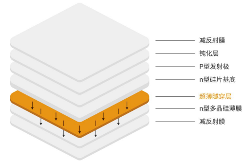
TOPCON电池结构
