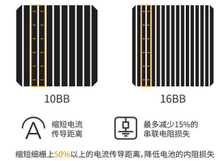
缩短细栅上50%以上的电流传导距离,降低电池的内阻损失
